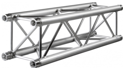
Poutre Carrée Litec Section heavy 30cm
